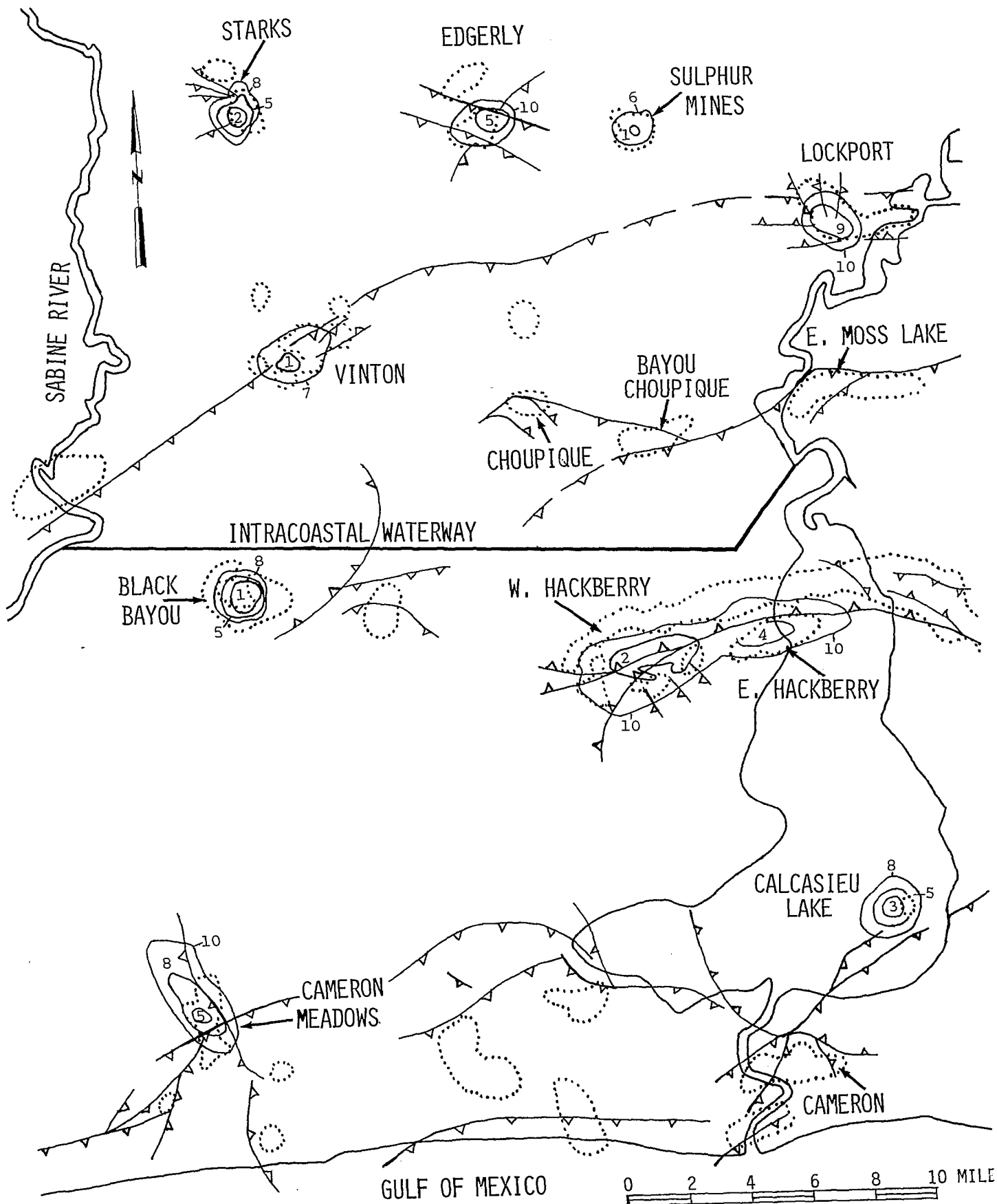
Figure B.3-34 Salt Fault Map (Wallace, 1966) B.3-104
